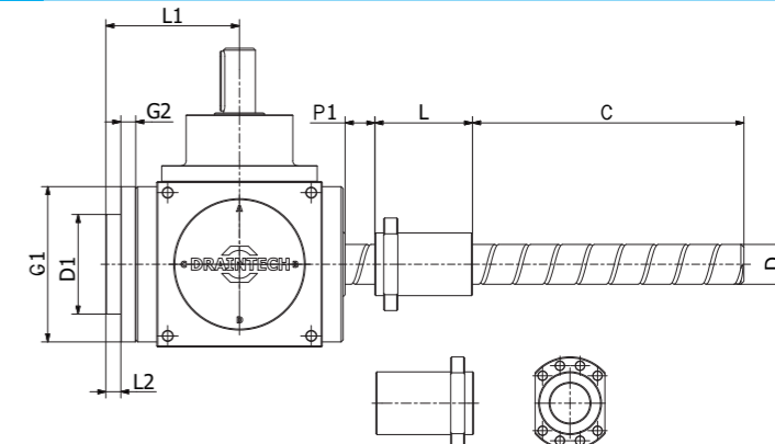
POSSIBILI SENSI DI MONTAGGIO DELLA CHIOCCIOLA
