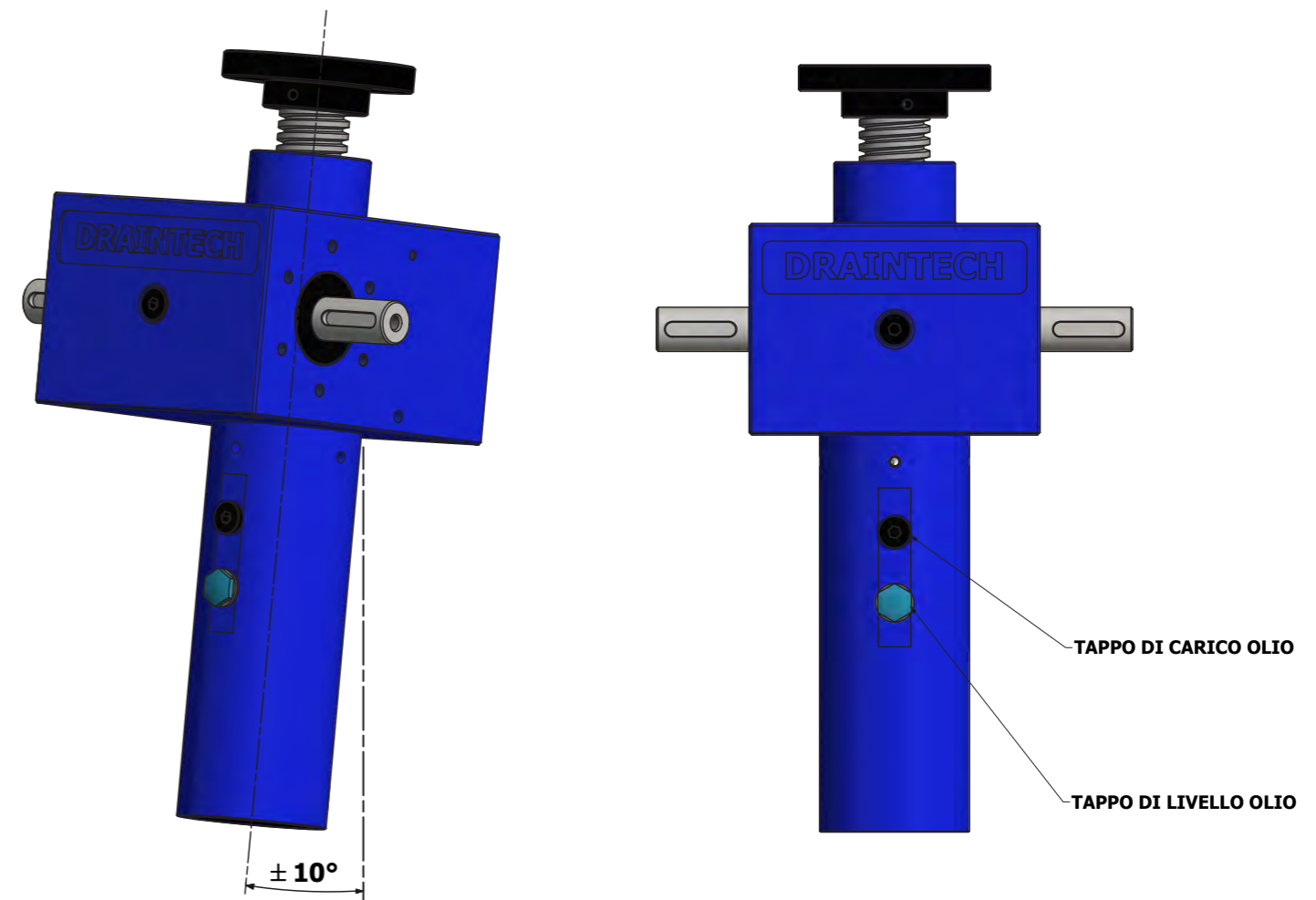
MONTAGGIO VERTICALE INCLINAZIONE MASSIMA AMMISSIBILE ± 10°
