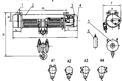
13.8 Электрическая таль CD1 10 т, 6 - 30 м с жестким креплением
