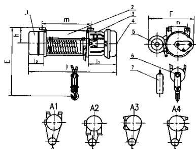
13.6 Электрическая таль MD1 0.5 - 5 т, 6 - 30 м с жестким креплением
