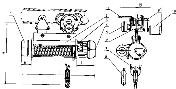
13.5 Электрическая таль MD1 0.5-5 т, 6-12 м
