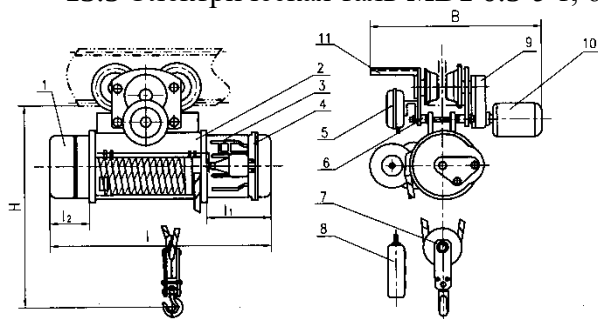
13.5 Электрическая таль MD1 0.5-5 т, 6-12 м
