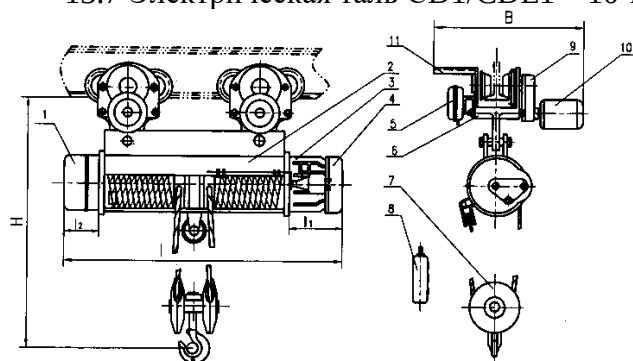
13.7 Электрическая таль CD1/CDL1 10 т, 6-30 м
