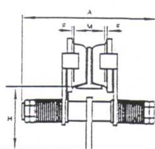
НЕПРИВОДНАЯ КОВКА
