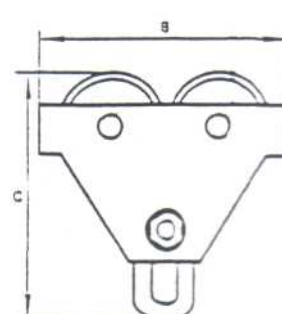
НЕПРИВОДНАЯ КОВКА
