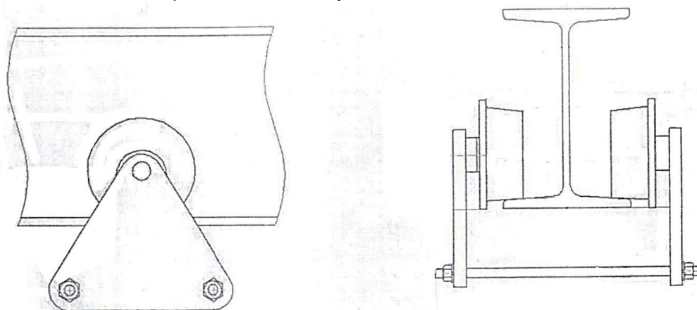
Рис. 2. Холостая тележка
